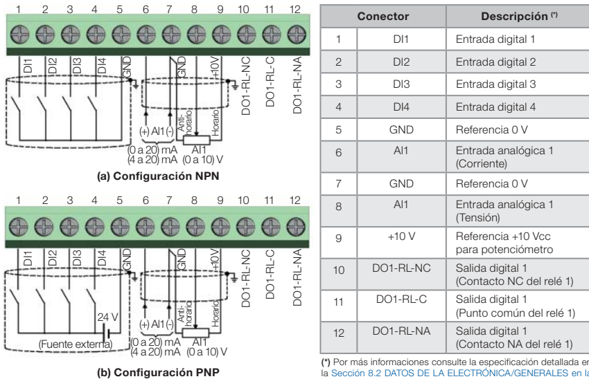
Figura 3.3: (a) y (b) Señales del conector de la tarjeta de control C300
