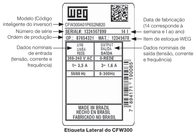
Figura 2.4: Descrição da etiqueta de identificação no CFW300
