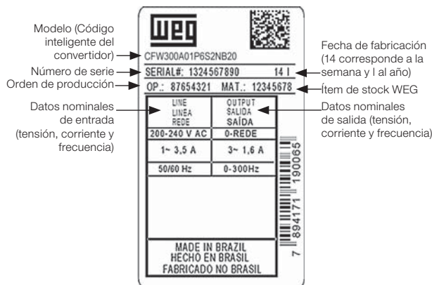
Etiqueta Lateral del CFW300
