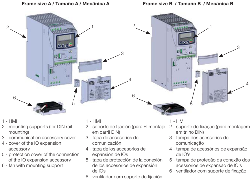
Figure A1: Main components of the CFW300 Figura A1: Principales componentes del CFW300 Figura A1: Componentes principais do CFW300
