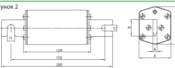
Габаритні розміри (мм)
