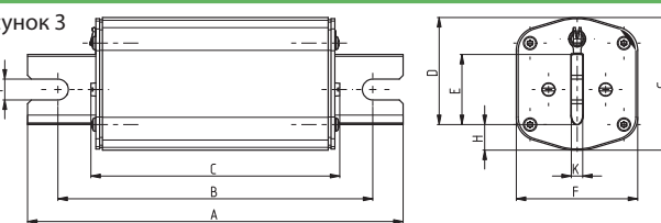
Габаритні розміри (мм)
