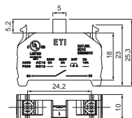
Блок контактів гвинтовий
