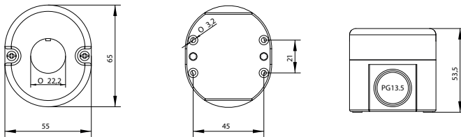
Корпус 2-місний
