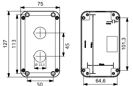
Корпус 2-місний
