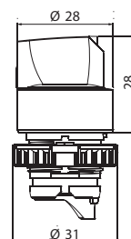
Вимикач-модуль двопозиційний „0-1”, трипозиційний „1-0-2”
