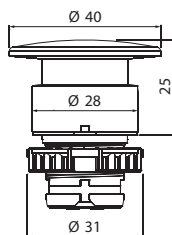
Кнопка-модуль „грибок” Ø 40 мм (із підсвічуванням)
