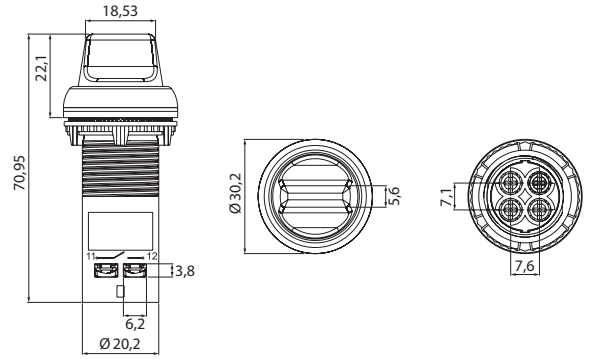
Вимикач "0-1" / Перемикач "1-0-2" моноблочний (із ключем)
