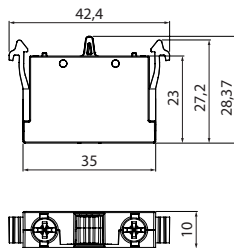
Блок контактів
