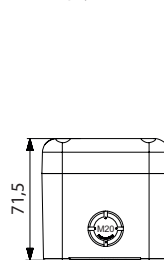
Корпус 4-місний
