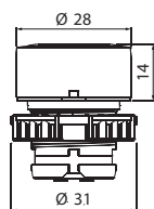
Кнопка-модуль заглиблена
