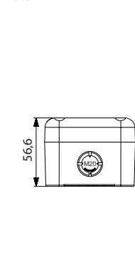
Корпус 3-місний
