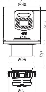
Кнопка-модуль „грибок” Ø 40 мм (із ключем)
