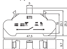
Блок контактів пружинний
