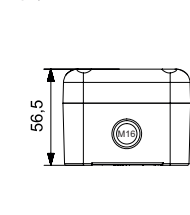
Корпус 1-місний
