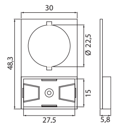
Шильд під маркувальну пластину
