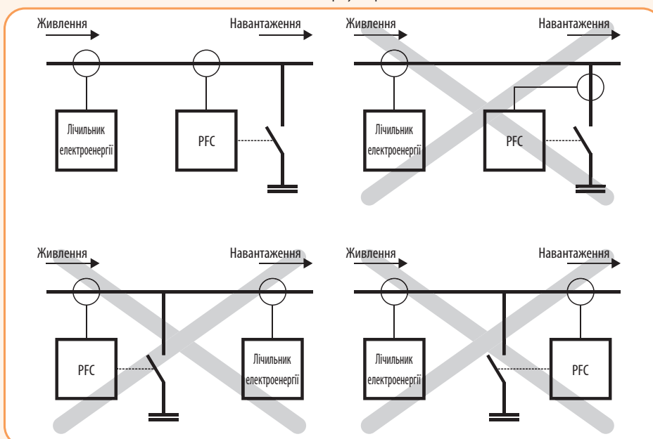
Установка регулятора
