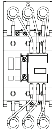
CEM 32... 80CN
