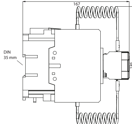
CEM 32... 80CN
