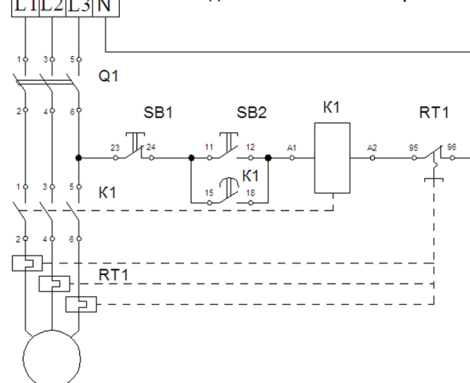
Схема підключення теплового реле
