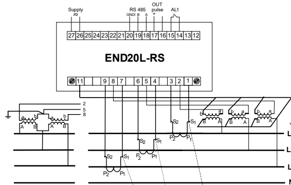
Непряме підключення до трифазної мережі
