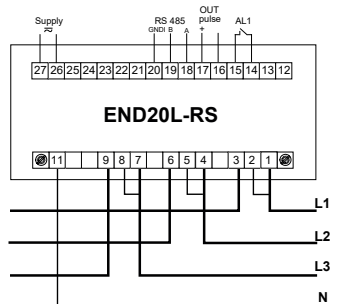
Пряме підключення до трифазної мережі
