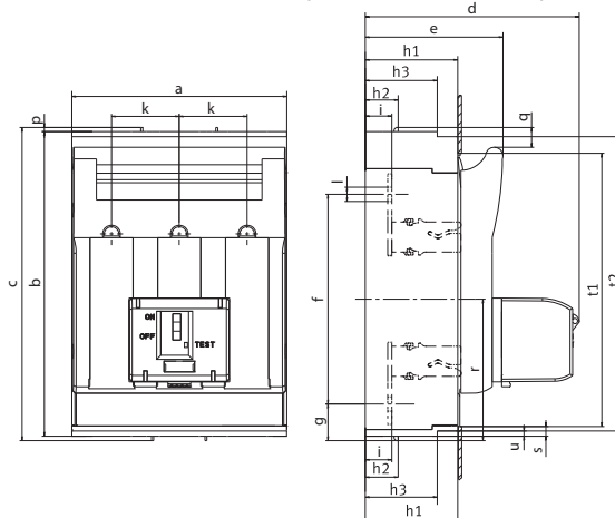
KVL 1, 2, 3 3p + MPFMU KVL-1, 2, 3 3p
