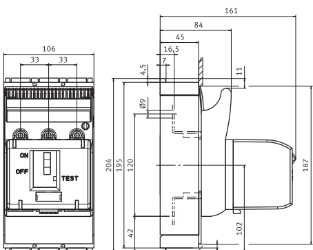
KVL 00 3p + MPFMU KVL-00 3p
