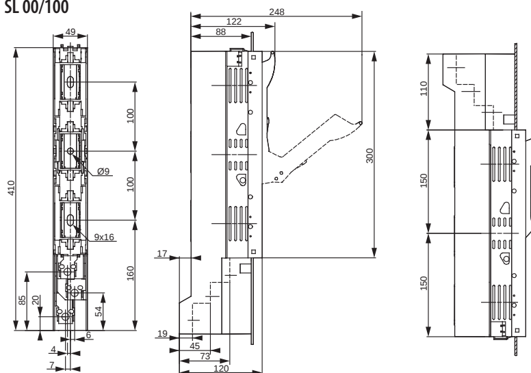
SL 00/100
