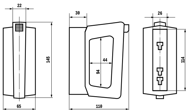
VRRN 00-3
