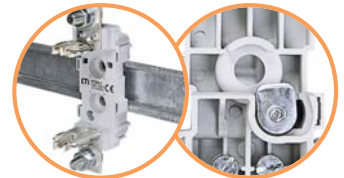
MS PT 00-1-2-3
