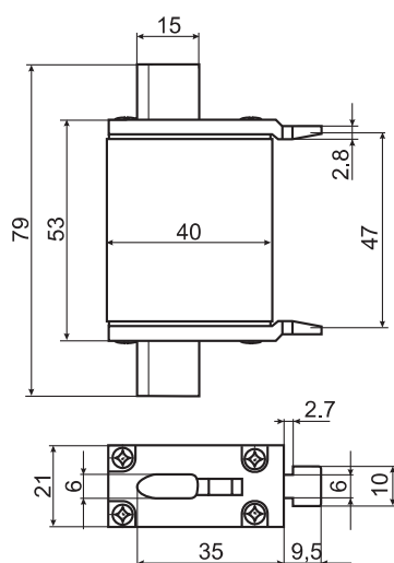
NV/NH 000 I
