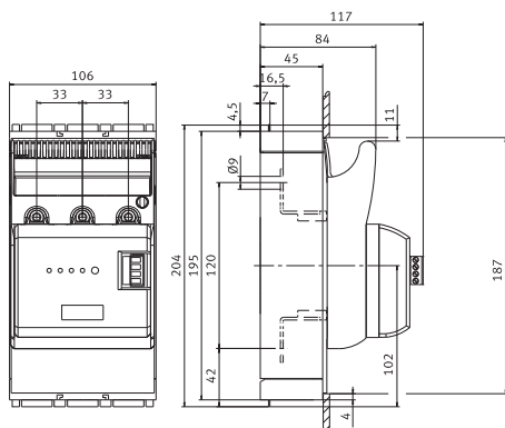
KVL 00 3p + MPFMU KVL-00 3p
