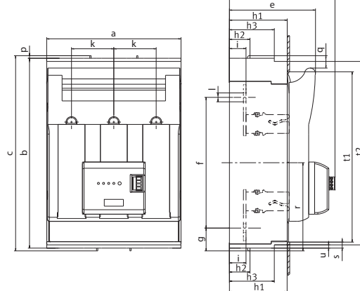
KVL 1, 2, 3 3p + MPFMU KVL-1, 2, 3 3p
