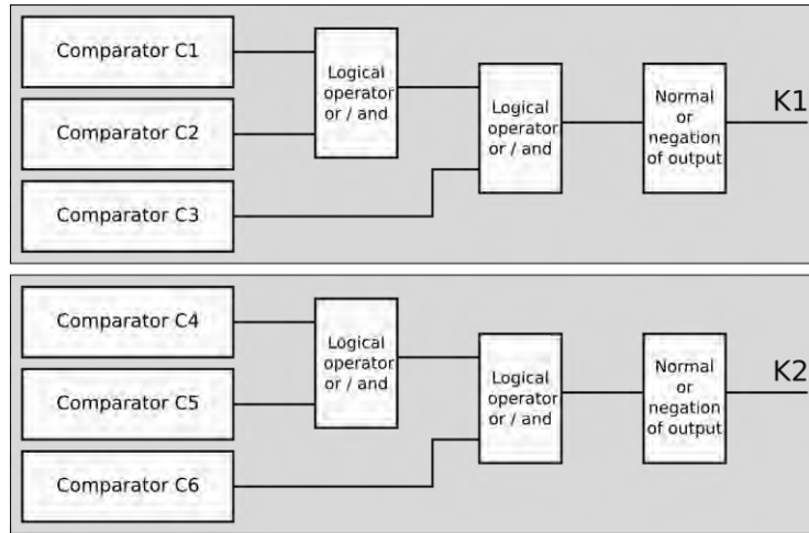
Рис.9. Компараторы и логические функции
