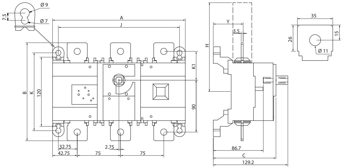
Тип корпусу B4T
