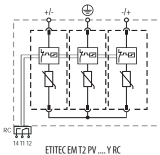
ETITEC EM T2 PV ... Y RC
