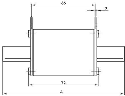
НН0, NH 1C
