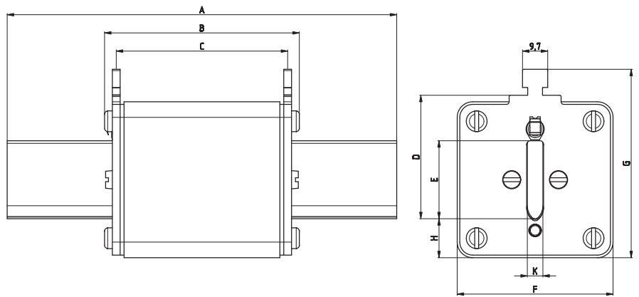
NH3 з візуальним індикатором спрацьовування зверху
