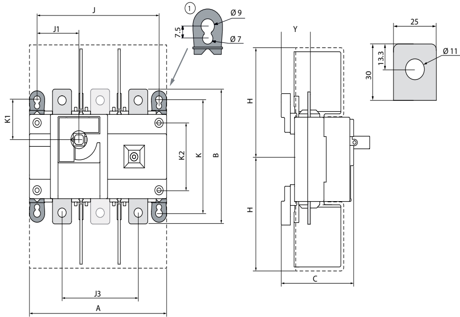
Тип корпусу B4
