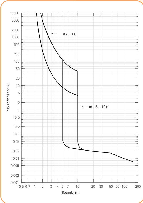
NBS-TMD 630/3 (500, 600A) Характеристика t-I
