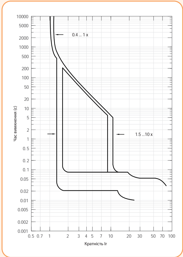
NBS-E (100 - 630A) Характеристика t-I
