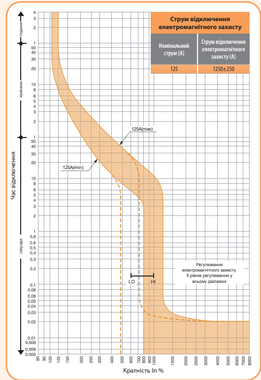
EB2 125 (125A) Характеристика t-I
