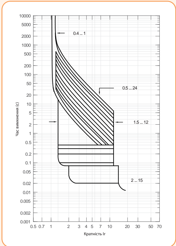
NBS-E&EC LCD (100 - 630A) Характеристика t-I
