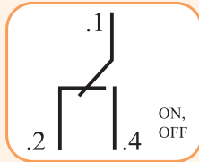
Схема, функція
