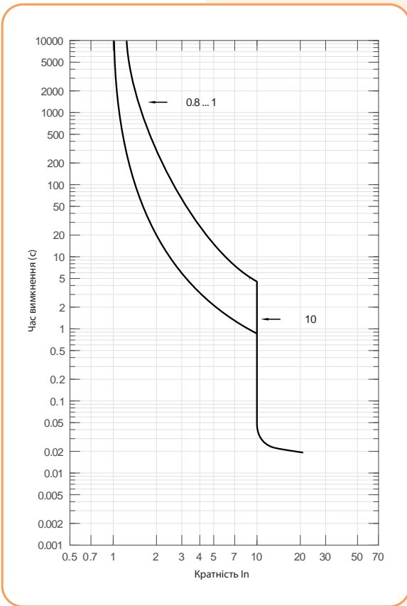
NBS-TMS 100/3 (32, 40A) Характеристика t-I
