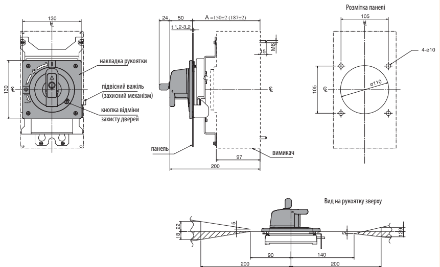
Рукоятка для ETIBREAK2 400&630 (монтаж на автоматичному вимикачі)
