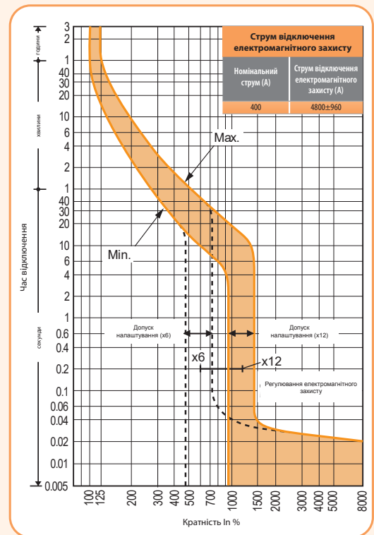
EB2 400 SF Характеристика t-I
