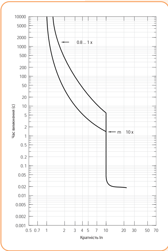
NBS-TMS 100/3 (20A) Характеристика t-I
