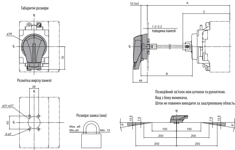
Рукоятка для ETIBREAK2 160&250 (монтаж на дверцята шафи)
