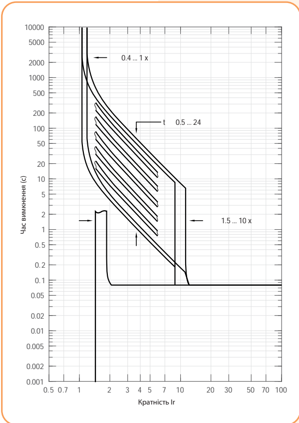
NBS-E (800 - 1600A) Характеристика t-I
