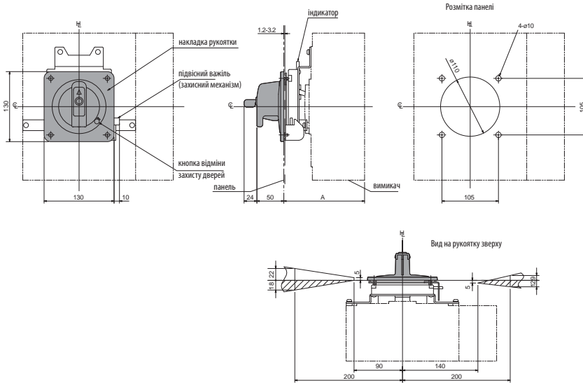
Рукоятка для ETIBREAK2 800&1000 (монтаж на автоматичному вимикачі)
