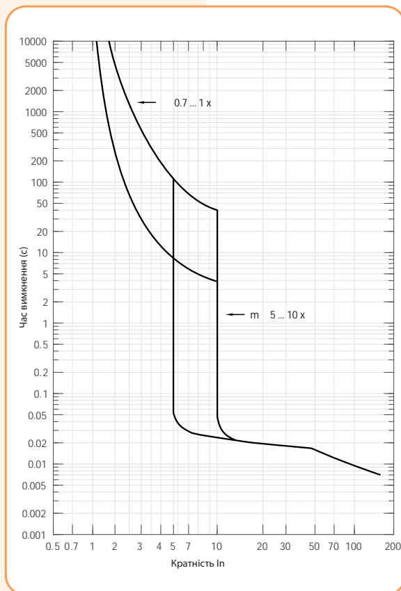
NBS-TMD 400/3 (315, 400A) Характеристика t-I
