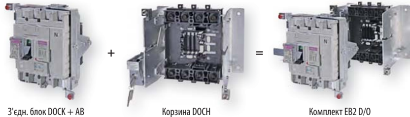
З'єдн. блок DOCK + АВ
